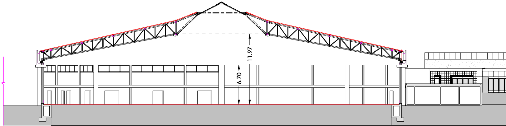
SEZIONE A-A
